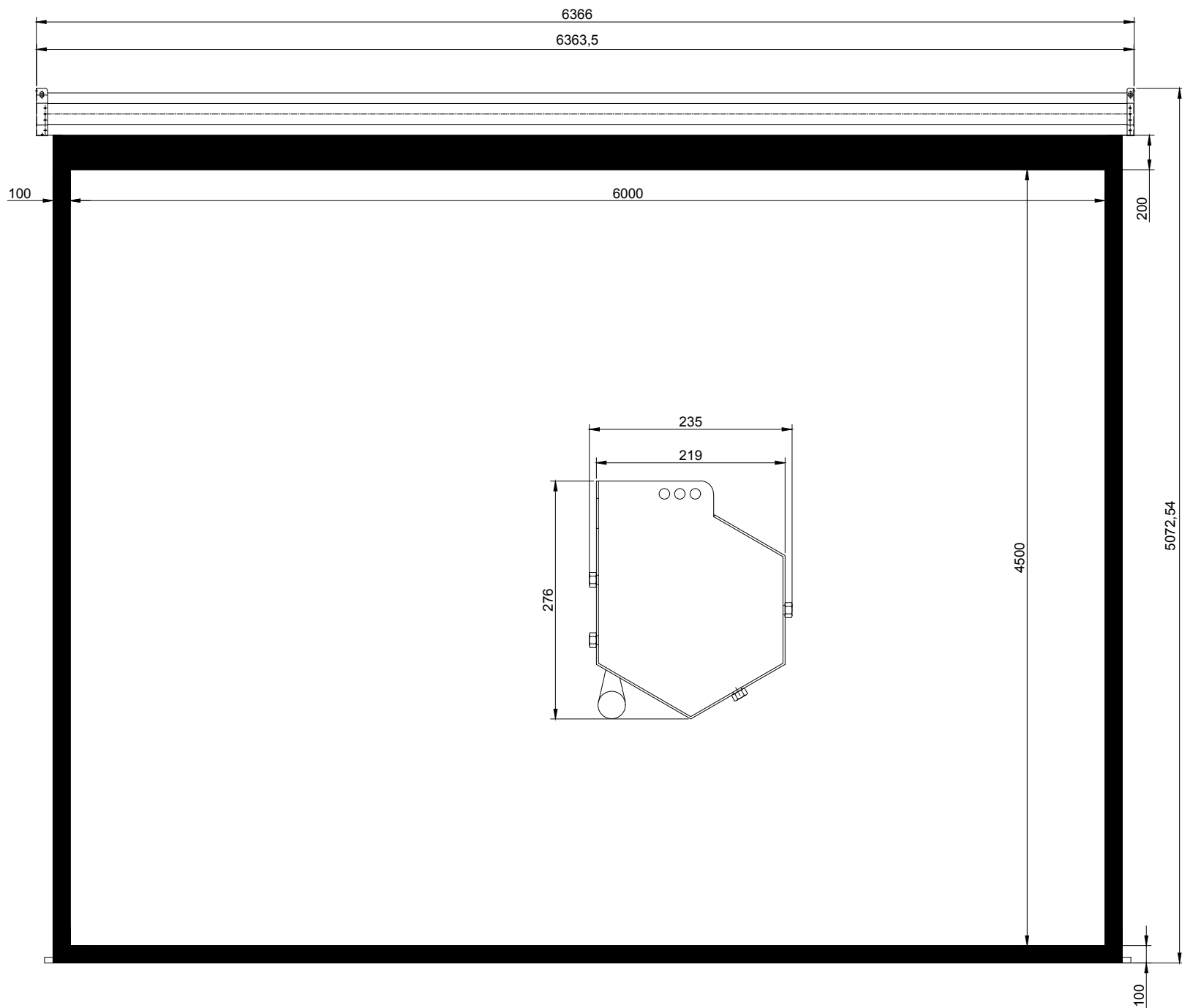
Classic Lyra (4:3) 630x480 (E 600x450/3 MW-S5/W) –электрический экран с БЕСШОВНЫМ полотном и ExtraDrop 20 см
